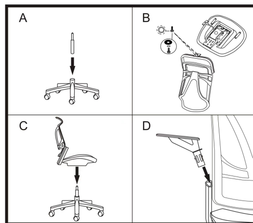
装配图
